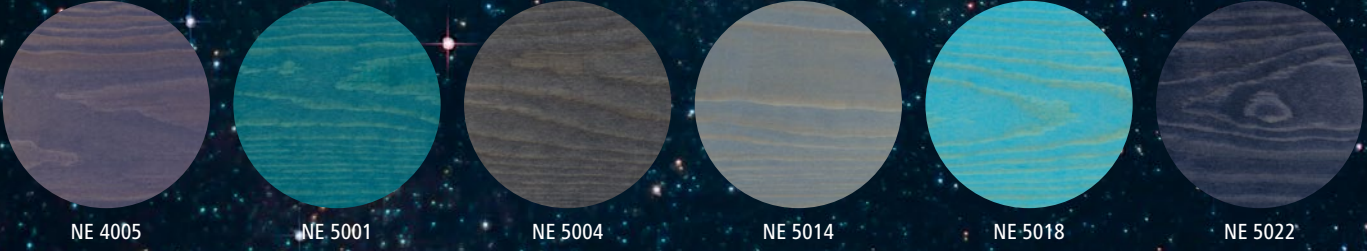
НЕПТУН
