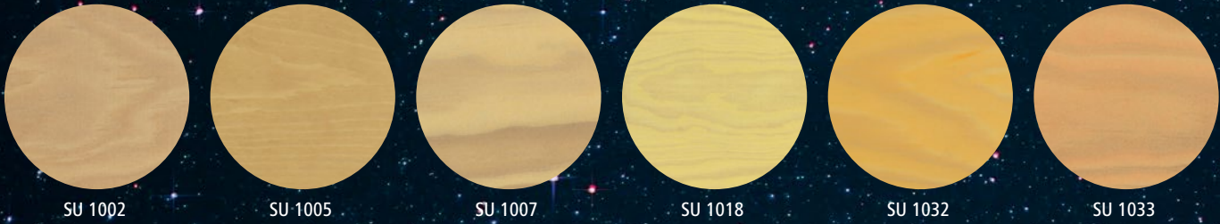
СОЛНЦЕ
