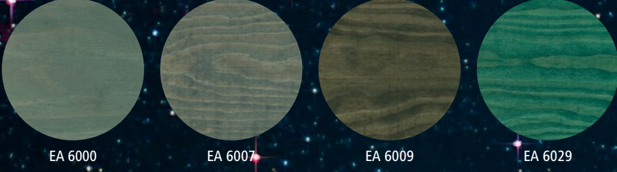
ЗЕМЛЯ
