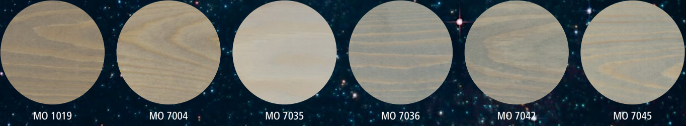
ЛУНА
